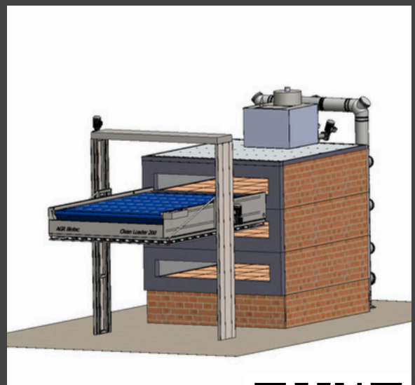
Belader entwickelt für AGR - Holzbacköfen mit integriertem Ascheabsaugsystem.
